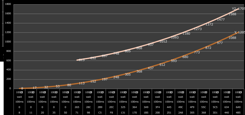
アクセル踏込量とモーターアシストカ (サンプル)
